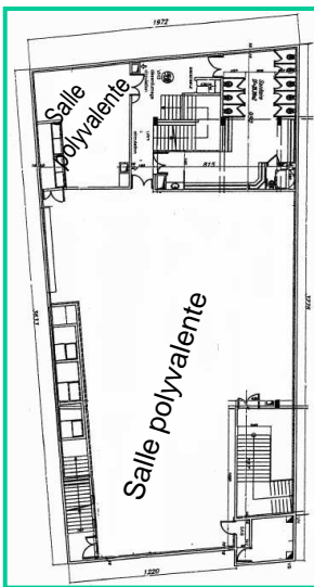
Sous-sol
